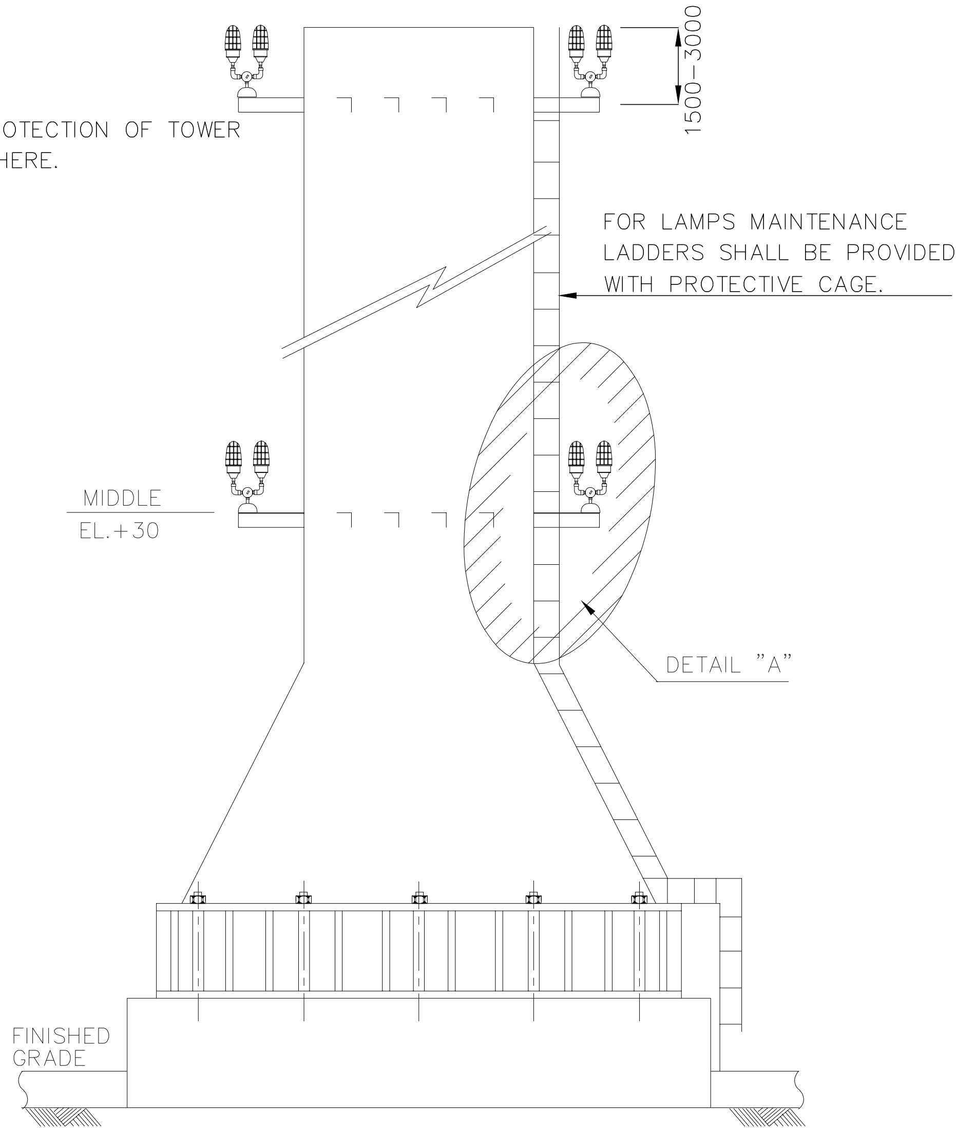
ELEVATION
