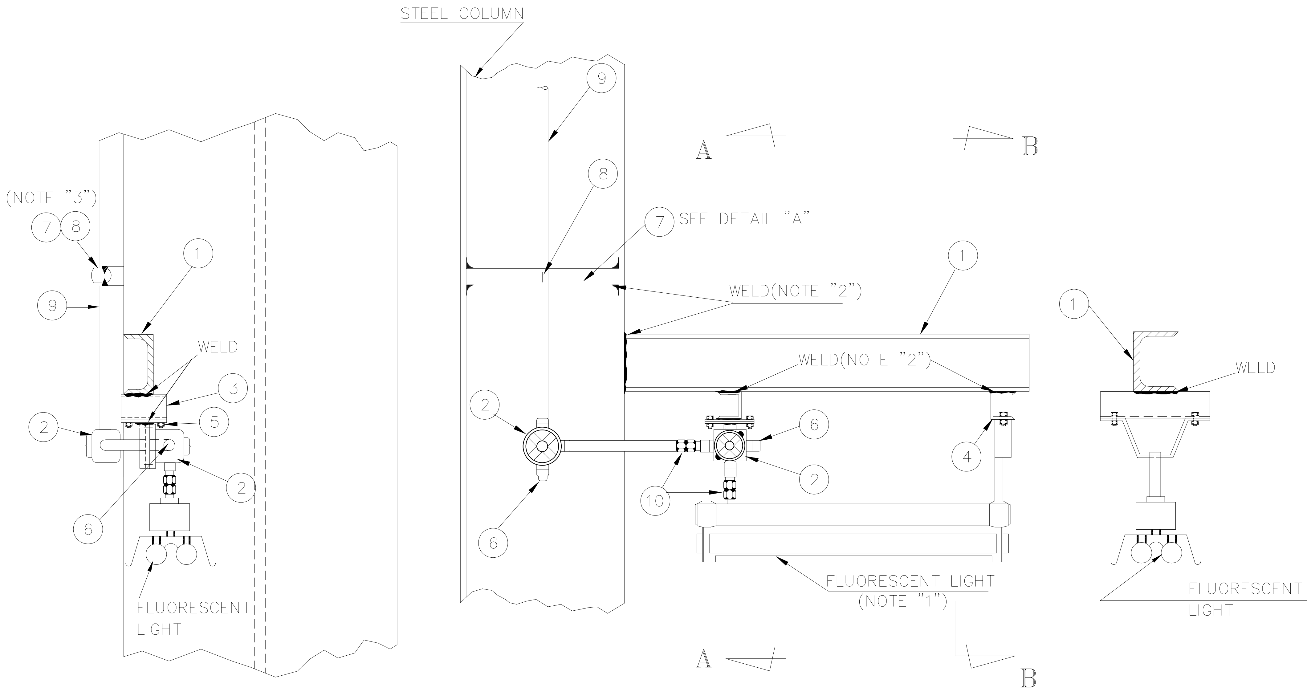
SECTION A-A
